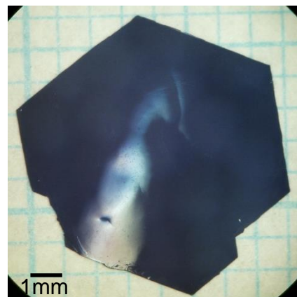
LiCoO 2
